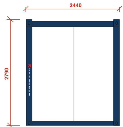
Elevación Este
