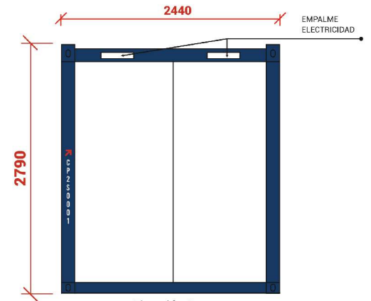
Elevación Oeste
