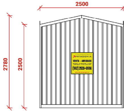
Elevación Oeste
