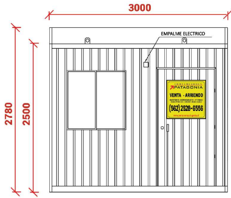
Elevación Sur
