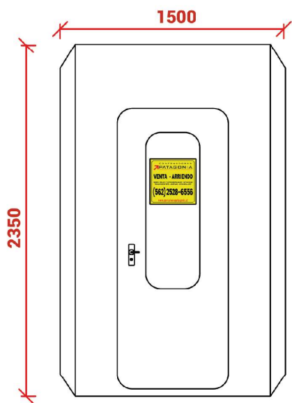
Elevación Oeste
