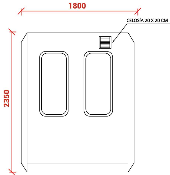
Elevación Sur
