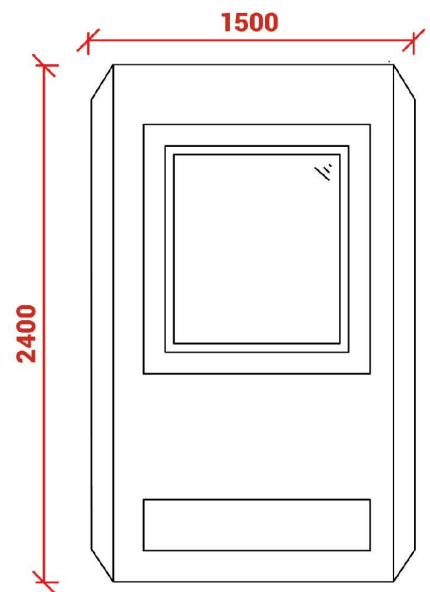
Elevación Sur
