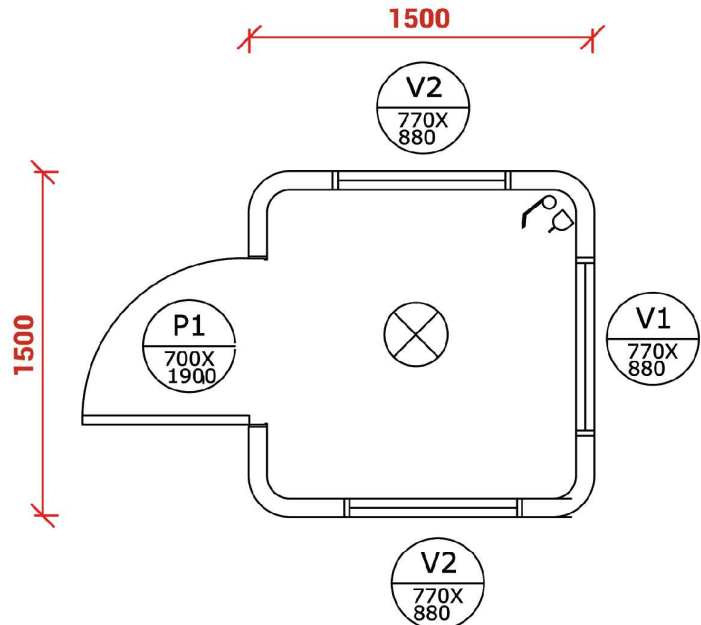
Planta
