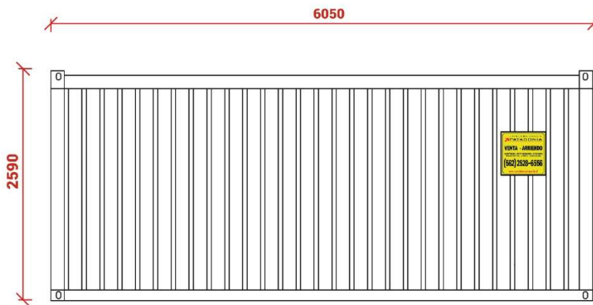
Elevación Norte
