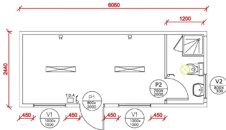
Planta
