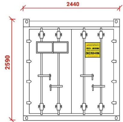
Elevación Oeste
