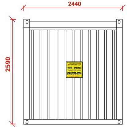
Elevación Oeste
