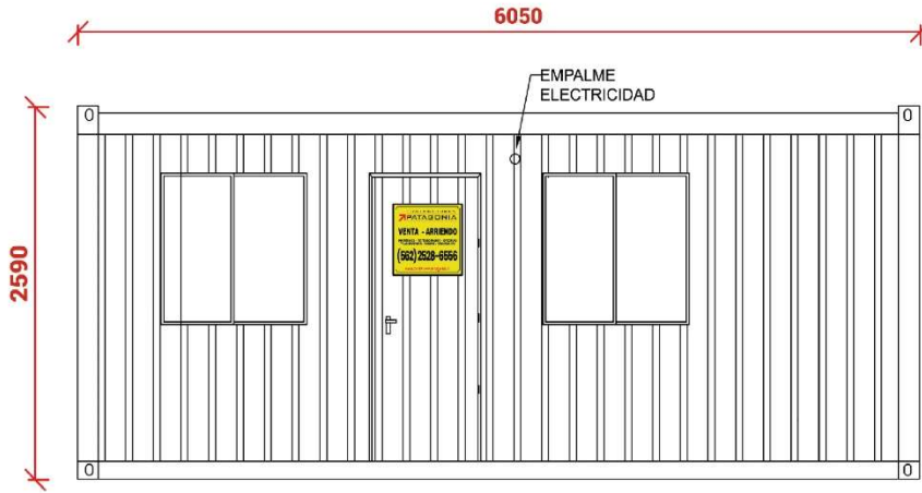
Elevación Sur
