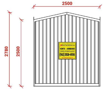
Elevación Oeste
