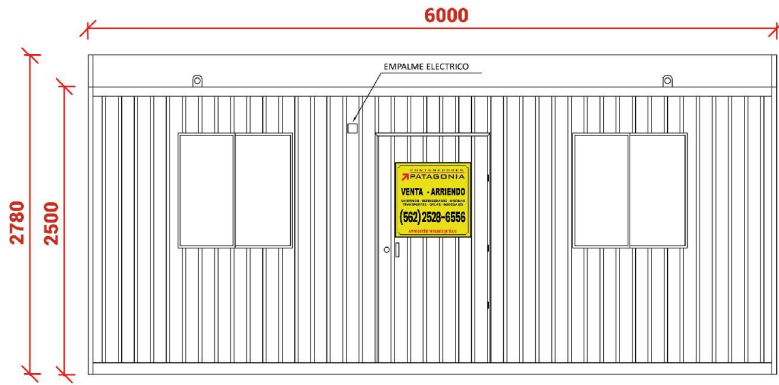
Elevación Sur
