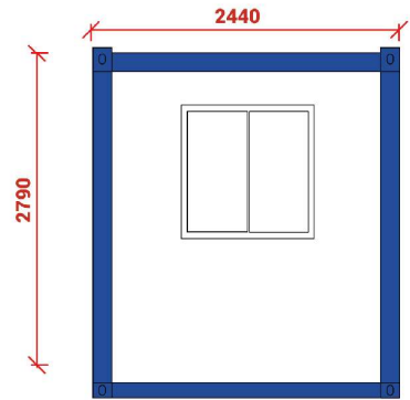
Elevación Este
