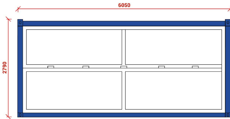
Elevación Norte
