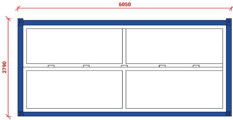
Elevación Sur
