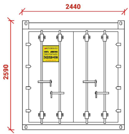
Elevación Este
