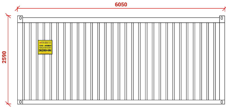
Elevación Sur
