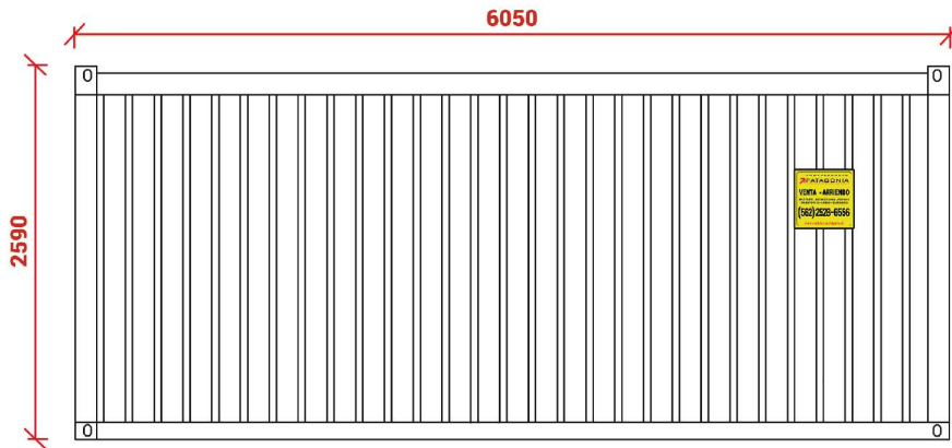
Elevación Norte
